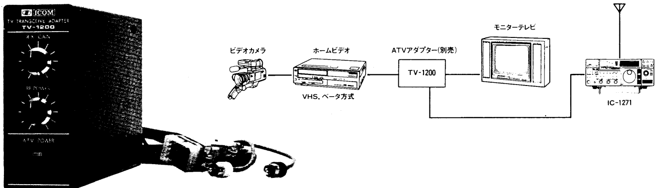
[送信系統概略図]
